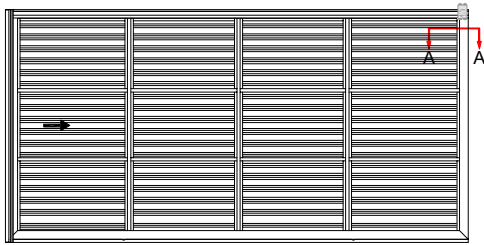
ΚΑΤΩΨΗ TOP VIEW
