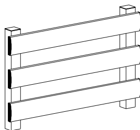
8 Εξωτερικό γραμμωτό ραμποτέ με ένθετο τζάμι 6 mm Patterned rabote with glass 6 mm
